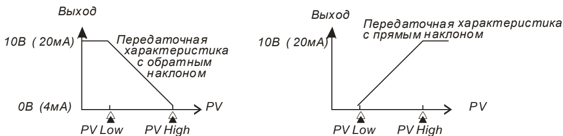
Рис 7: Пропорциональный выход
