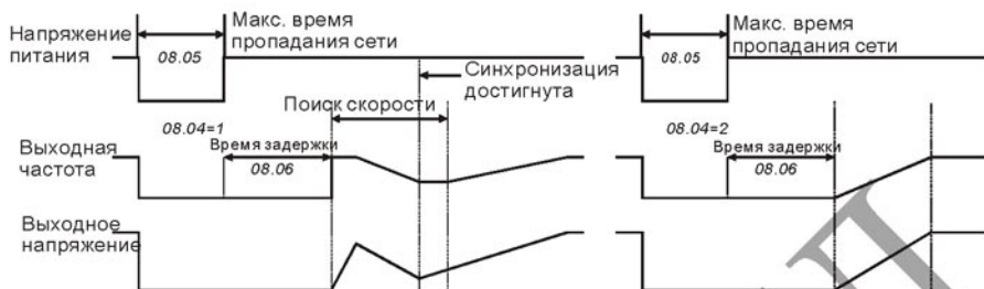
Рестарт после пропадания напряжения питания
