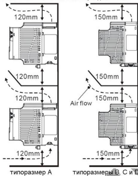
Установка с металлическим разделителем
