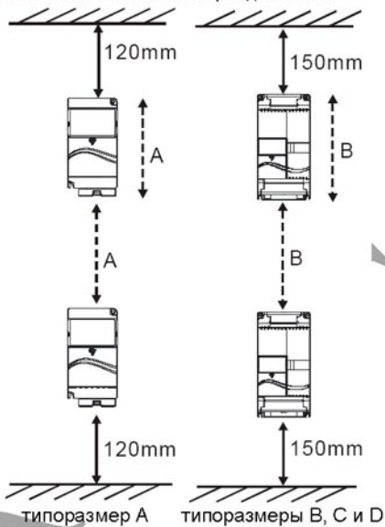
Установка без метал-го разделителя
